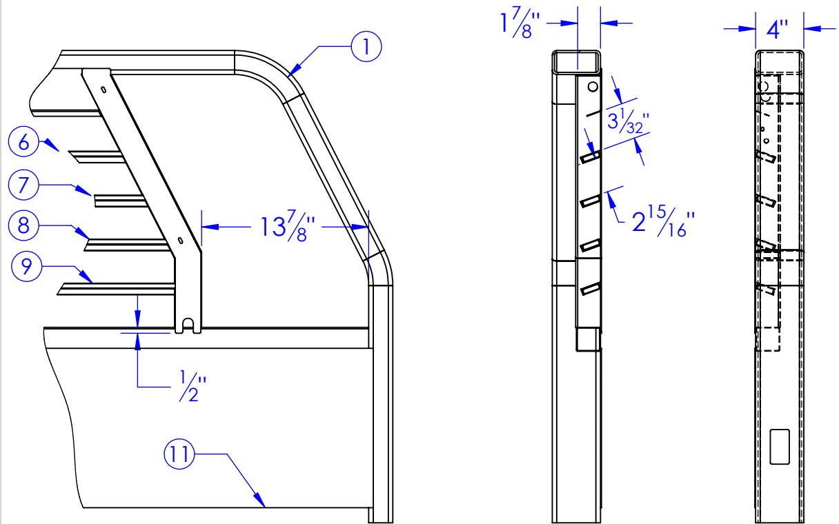
SECTION D-D
